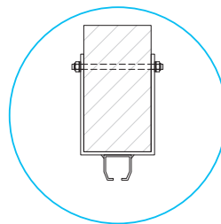
auf Holzbalken mit U-Bügel
