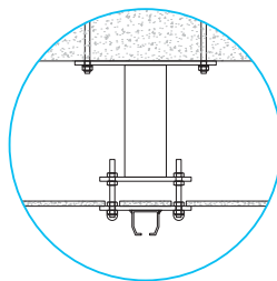
abgehängte Decke von 290-600 mm
