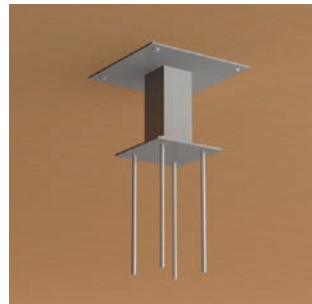
Unterkonstruktion für Deckenhaken - Montage auf Konstruktionsvollholzdecke
