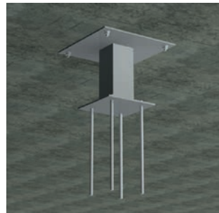
Unterkonstruktion für Deckenhaken - Montage auf Vollbetondecke
