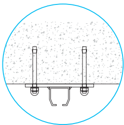
Direkt auf tragender Decke
