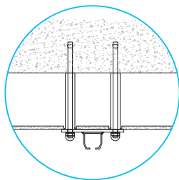
abgehängte Decke bis 290 mm
