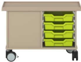
Bau- und Konstruktionstisch klein 444.013.207K L 82 x B 48,2 x H 55,5 cm
