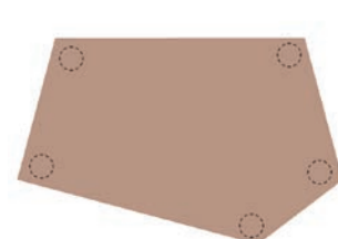
FORMA-Tisch fünfeckig groß Breite: 1764 mm Tiefe: 1122 mm TI260905
